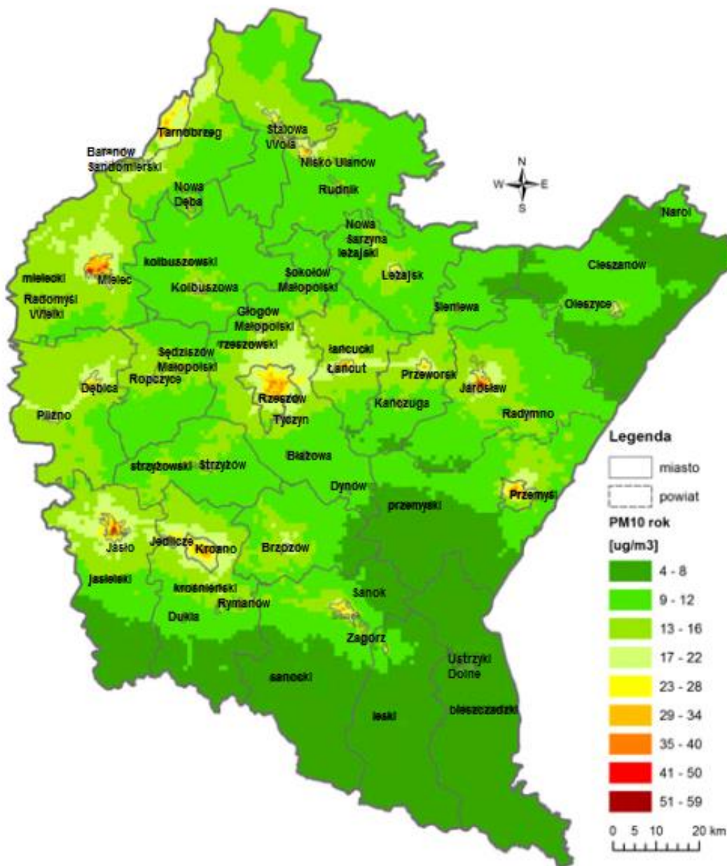
Mapa 8 Rozkład stężenia rocznego pyłu zawieszonego PM10 na terenie
