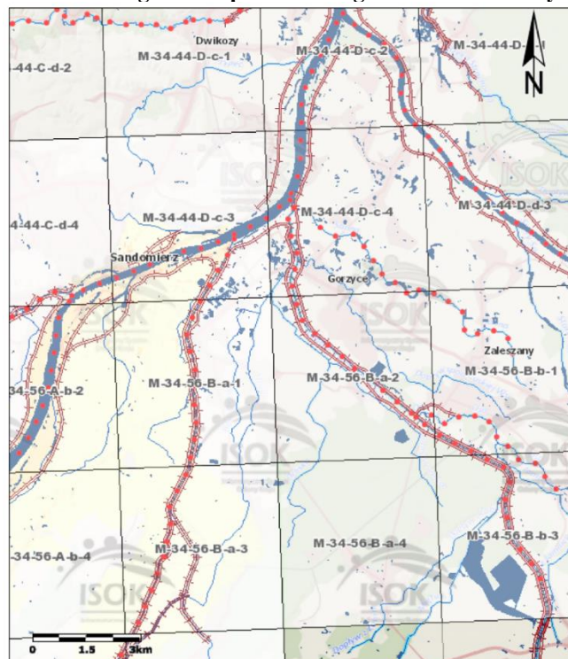
Mapa 11 Obszar zagrożenia powodziowego na terenie Gminy Gorzyce
