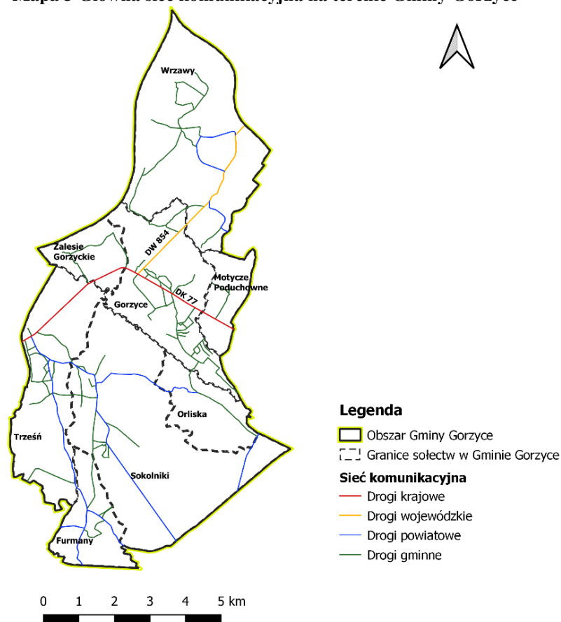
Mapa 3 Główna sieć komunikacyjna na terenie Gminy Gorzyce
